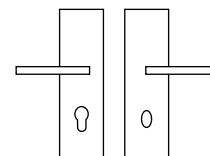
Cylindre euro avec bouton Profile cylinder with turn piece 05
